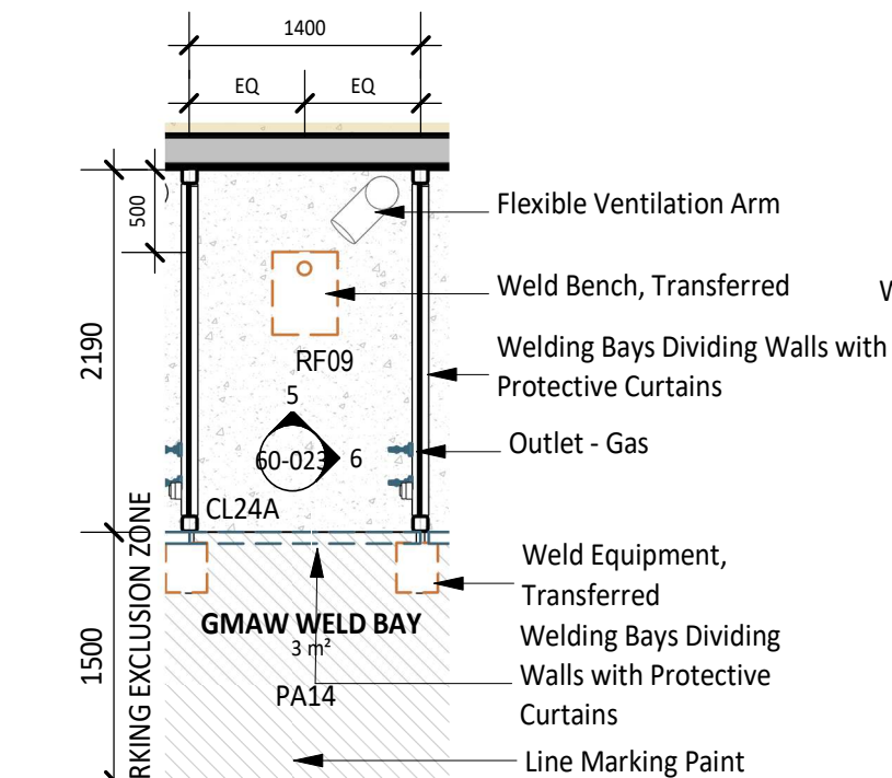
4 PLAN DETAIL 1 : 50
