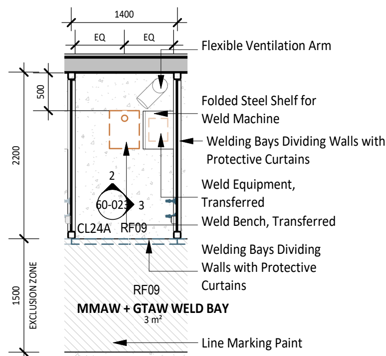
1 PLAN DETAIL 1 : 50
